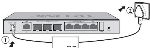
图3-3 电源连接示意图
