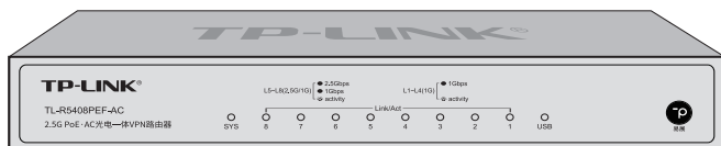
图1-1 TL-R5408PEF-AC前面板示意图
